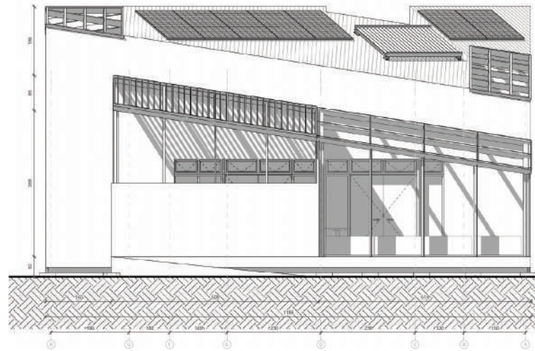
[18] Elevación frontal
