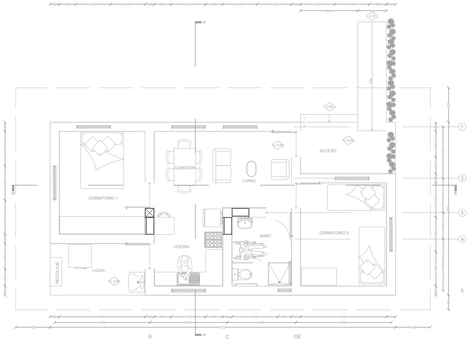
[53] Planta arquitectura
