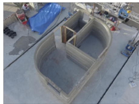
Imagen N°2: Construcción de casa impresa 3D. Fuente: Be-More, 2018.
